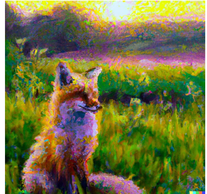
Dall-E 2.0
